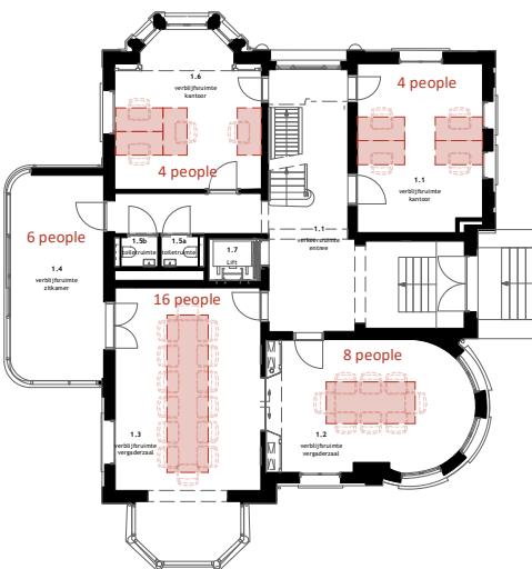
niveau 1 215m²
